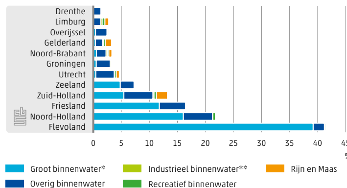
Aandeel binnenwater t.o.v. totale oppervlakte (excl. buitenwater) per provincie, 2010
