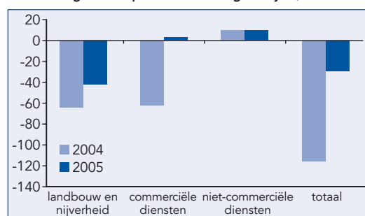
Figuur 1. Banen van werknemers, jaargemiddelden, veranderingen ten opzichte van voorgaand jaar, × 1000
