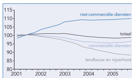
Figuur 2. Banen van werknemers, gecorrigeerd voor seizoen, 2001=100
