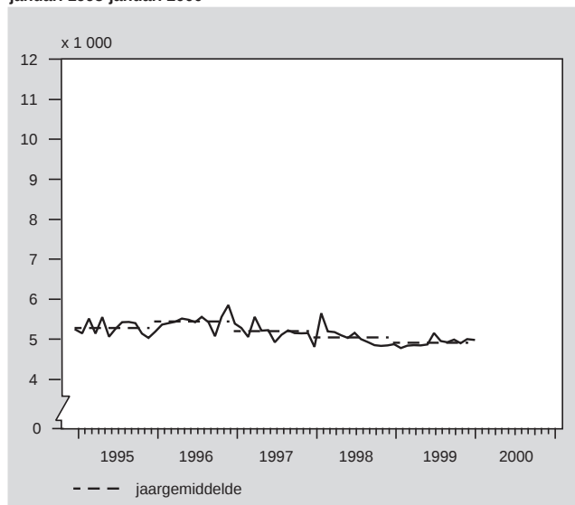
Emigratie per maand, gecorrigeerd voor seizoeninvloeden, januari 1995-januari 2000
