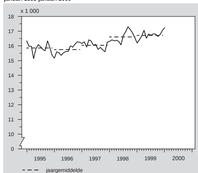
Levendgeborenen per maand, gecorrigeerd voor seizoeninvloeden, januari 1995-januari 2000
