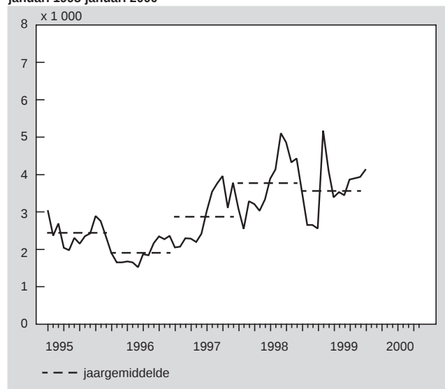
Asielzoekers per maand, januari 1995-januari 2000
