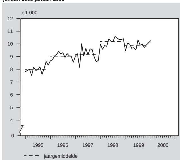
Immigratie per maand, gecorrigeerd voor seizoeninvloeden, januari 1995-januari 2000
