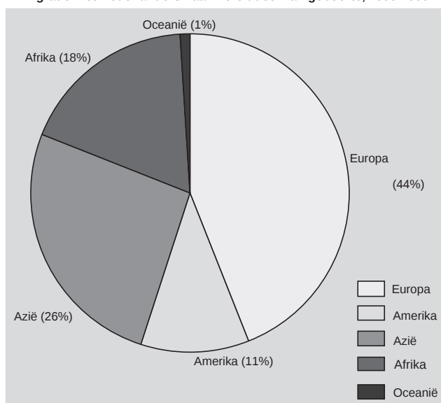
Immigratie niet-Nederlanders naar werelddeel van geboorte, 1995-1999
