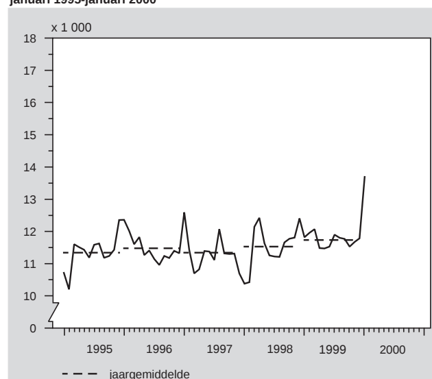
Overledenen per maand, gecorrigeerd voor seizoeninvloeden, januari 1995-januari 2000
