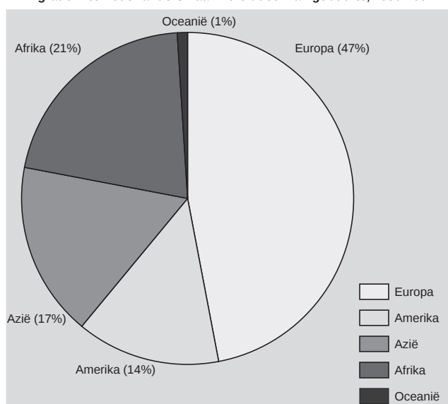
Immigratie niet-Nederlanders naar werelddeel van geboorte, 1990-1994
