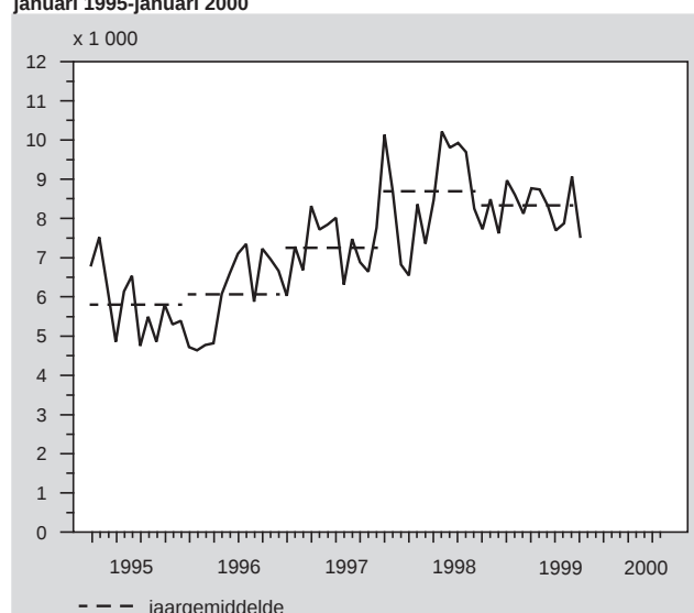
Bevolkingsgroei per maand, gecorrigeerd voor seizoeninvloeden, januari 1995-januari 2000
