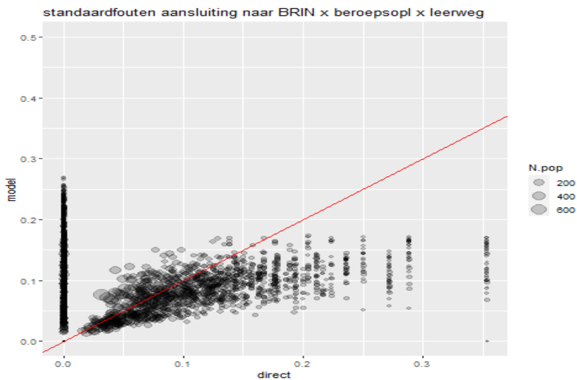
Figuur II.4 Standaardfouten voor modelgebaseerde en directe schattingen voor fracties aansluiting naar BRIN x beroepsopleiding x leerweg.
