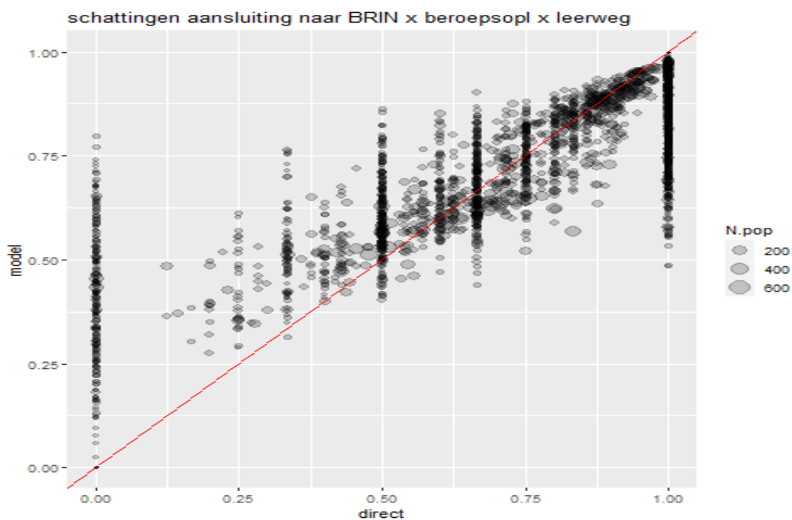
Figuur II.3 Modelgebaseerde en directe schattingen voor fracties aansluiting naar BRIN x beroepsopleiding x leerweg.
