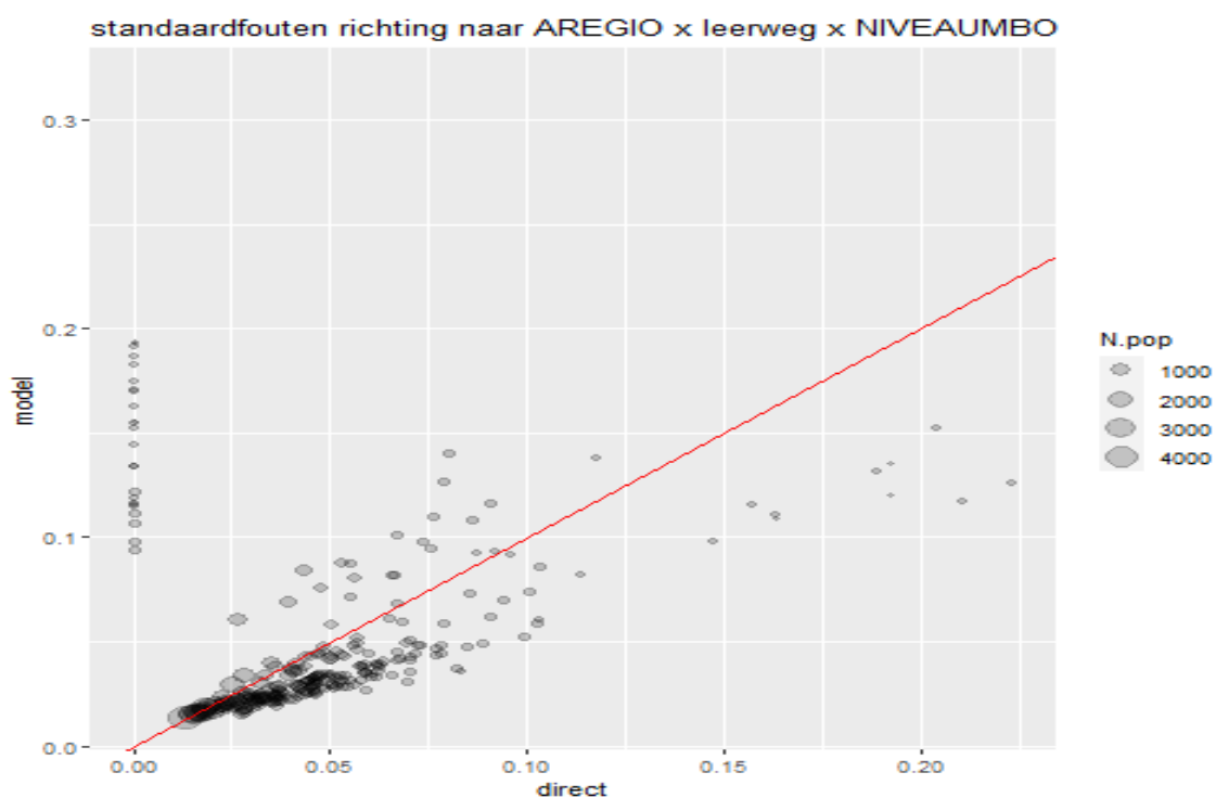
Figuur II.24 Standaardfouten voor modelgebaseerde en directe schattingen voor fracties richting naar Arbeidsmarktregio x leerweg x NIVEAUMBO .
