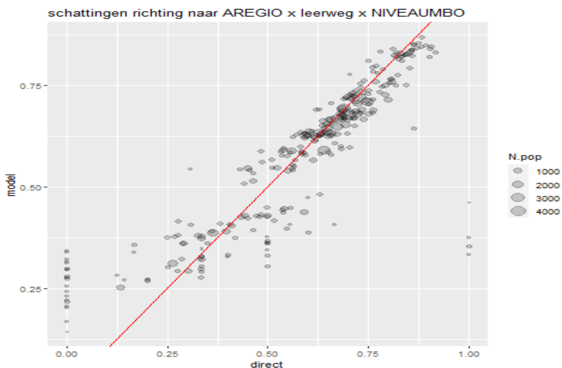
Figuur II.23 Modelgebaseerde en directe schattingen voor fracties richting naar Arbeidsmarktregio x leerweg x NIVEAUMBO .
