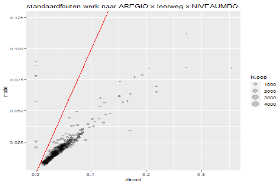
Figuur II.18 Standaardfouten voor modelgebaseerde en directe schattingen voor fracties werk naar Arbeidsmarktregio x leerweg x NIVEAUMBO .
