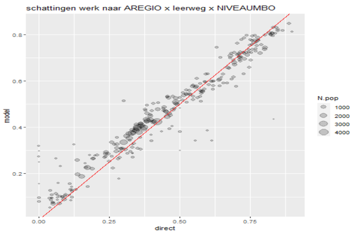
Figuur II.17 Modelgebaseerde en directe schattingen voor fracties werk naar Arbeidsmarktregio x leerweg x NIVEAUMBO .
