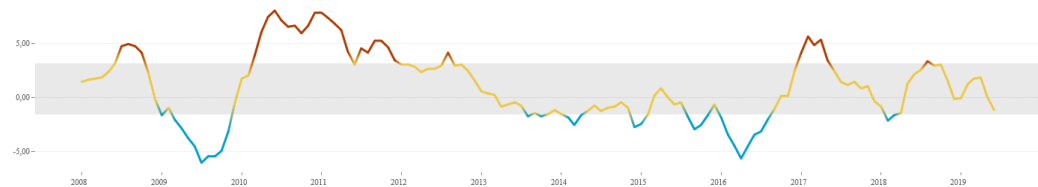
Invoer industriële producten (%-jaarmutatie)
