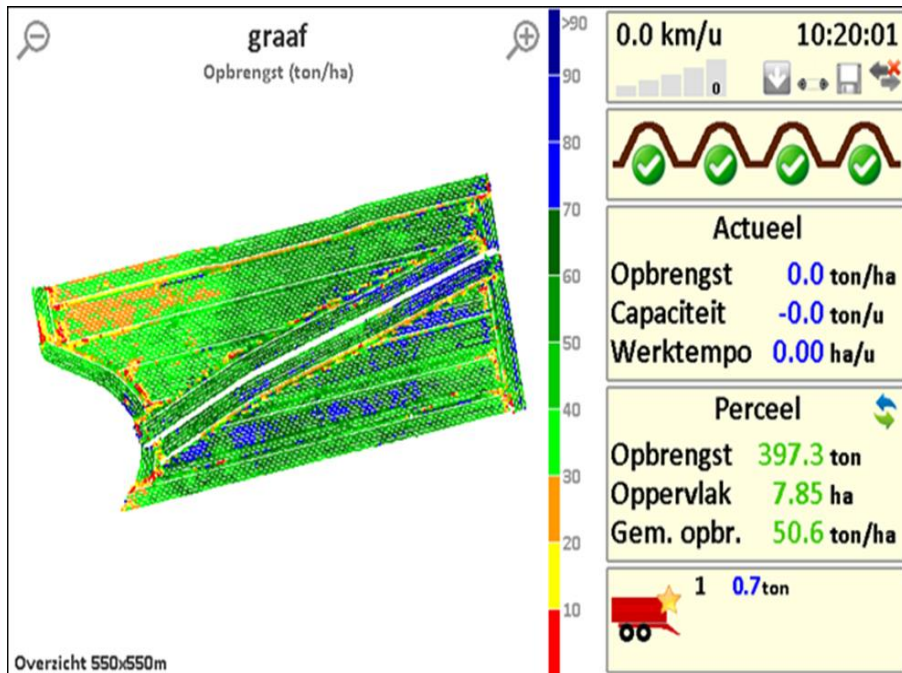
Display oogstmachine
