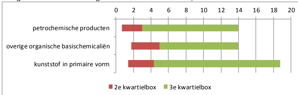
Figuur 3.16 Gehalte aan stikstof in afvalwater in µg per liter (alle stromen) voor enkele bedrijfsklassen binnen de bedrijfstak basischemicaliën in 2008, 2010 en 2012
