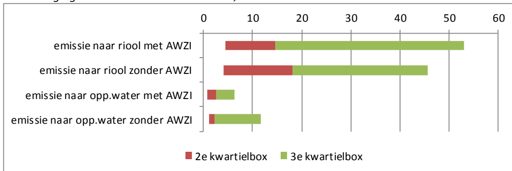
Figuur 3.15 Gehalte aan stikstof in afvalwater in µg per liter per afvalwaterstroom in de vervaardiging van basischemicaliën in 2008, 2010 en 2012
