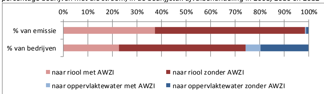
Figuur 3.10 Procentuele verdeling van emissiestromen van stikstof in afvalwater met het percentage bedrijven met die stroom, in de bedrijfstak afvalbehandeling in 2008, 2010 en 2012
